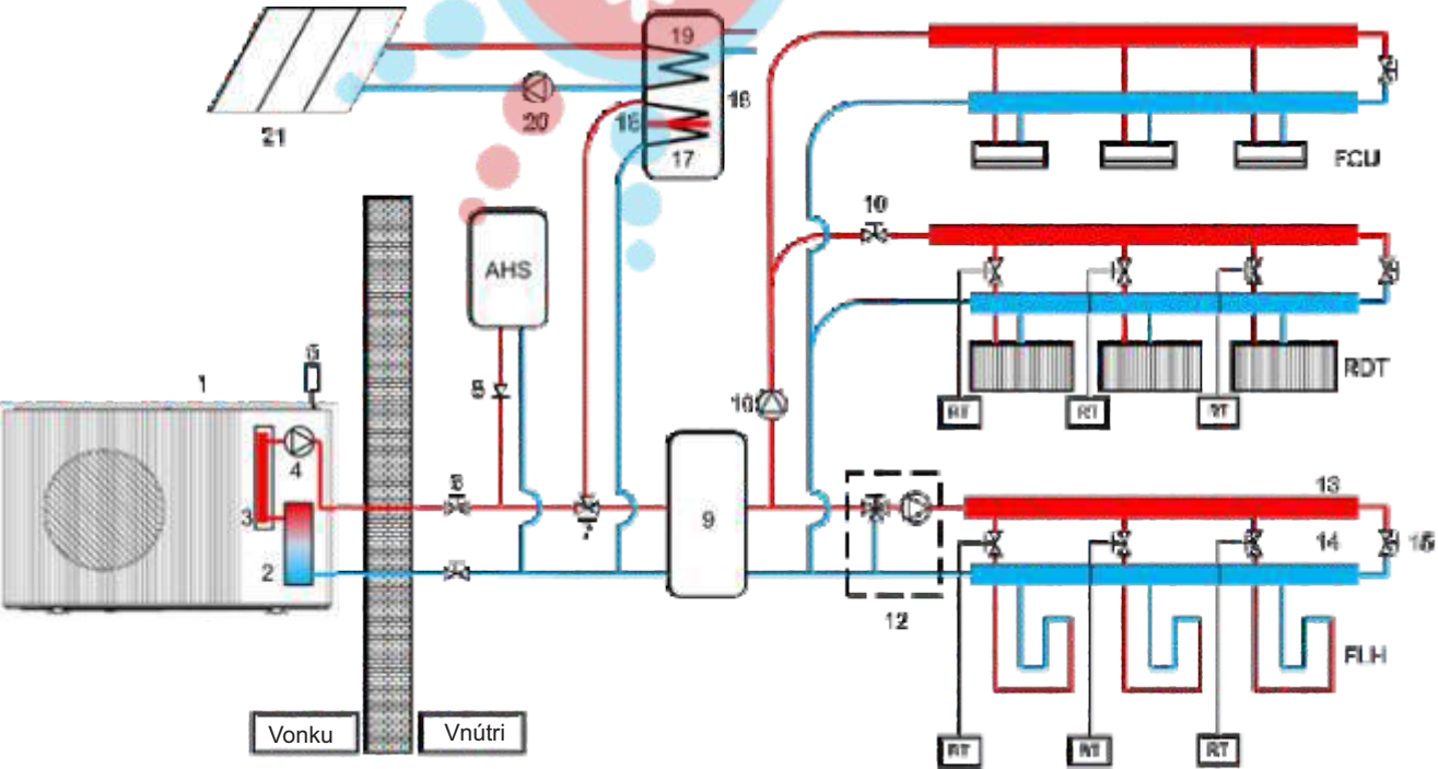
Obrázok 3.8: Vykurovanie s tepelným čerpadlom a AHS, chladenie tepelným čerpadlom a solárny ohrev vody
