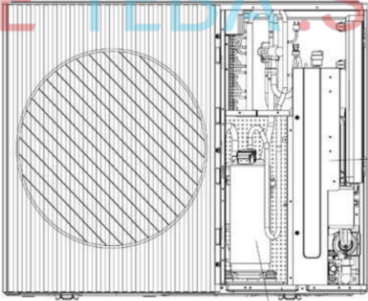
Chladivový systém
